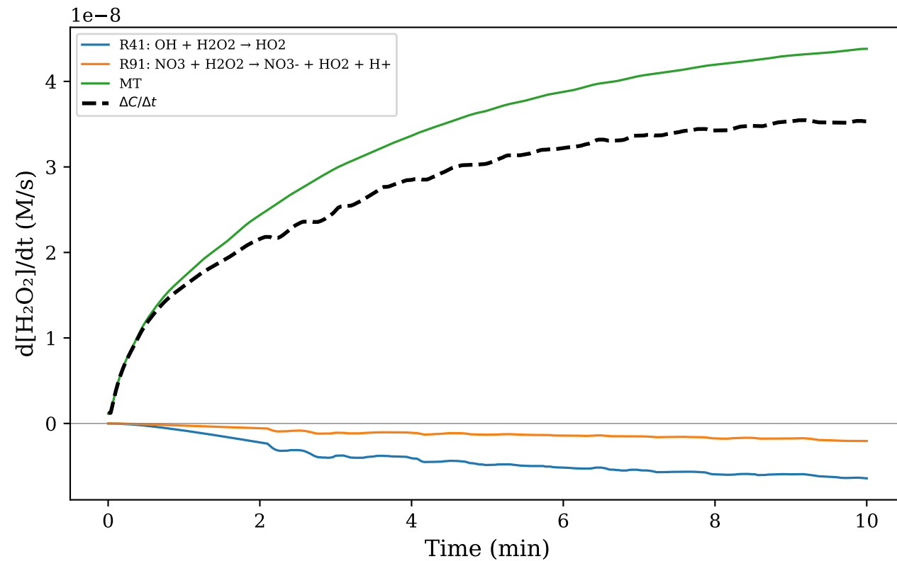
(d) \text{H}_2\text{O}_2
